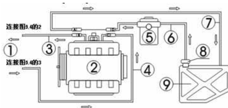
IMAGEN 6 Conexión de mangueras para Limpieza en-vehículo.
