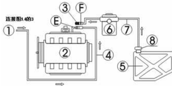
IMAGEN 7 Conexión de mangueras para limpieza en-vehículo
